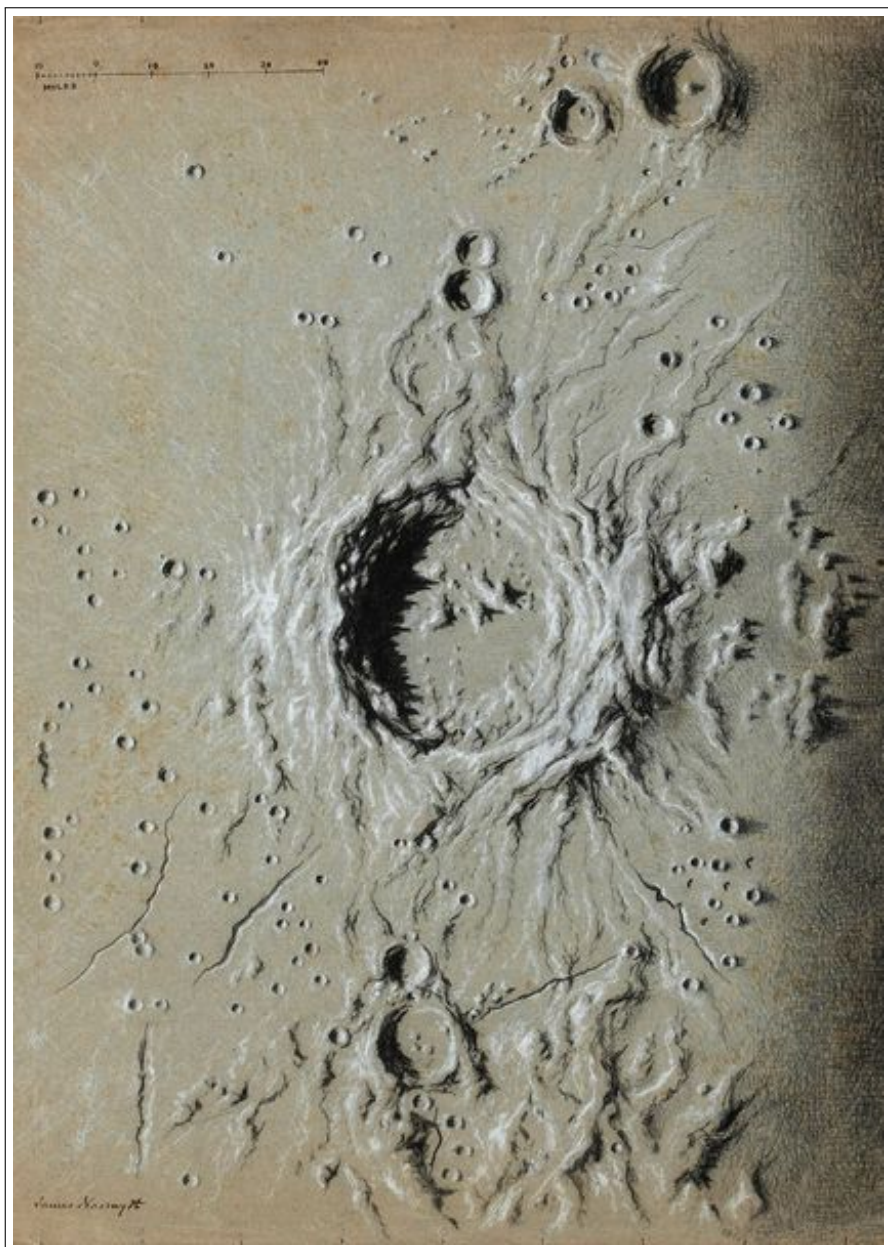
Dessin d'un cratère lunaire - James Nasmyth (1808-1890)
